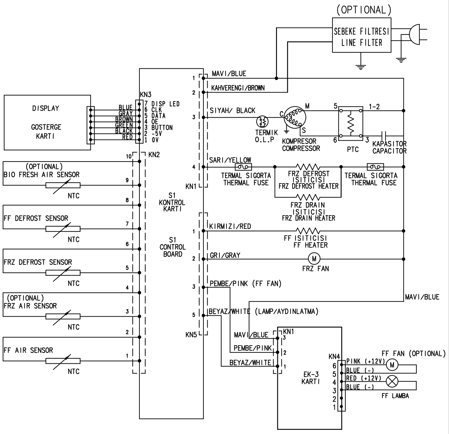
WIRING DIAGRAM ELEKTRİK DEVRE SEMASI
